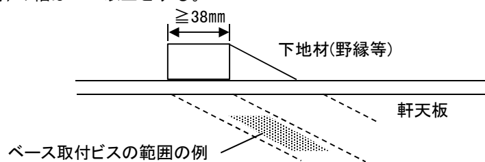
図2－下地材(野縁等)
