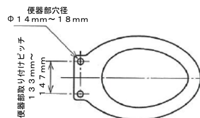
図2－JISに規定する洋風便器寸法
